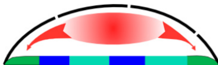
Схема заселения насекомыми коровьего помета. День третий
